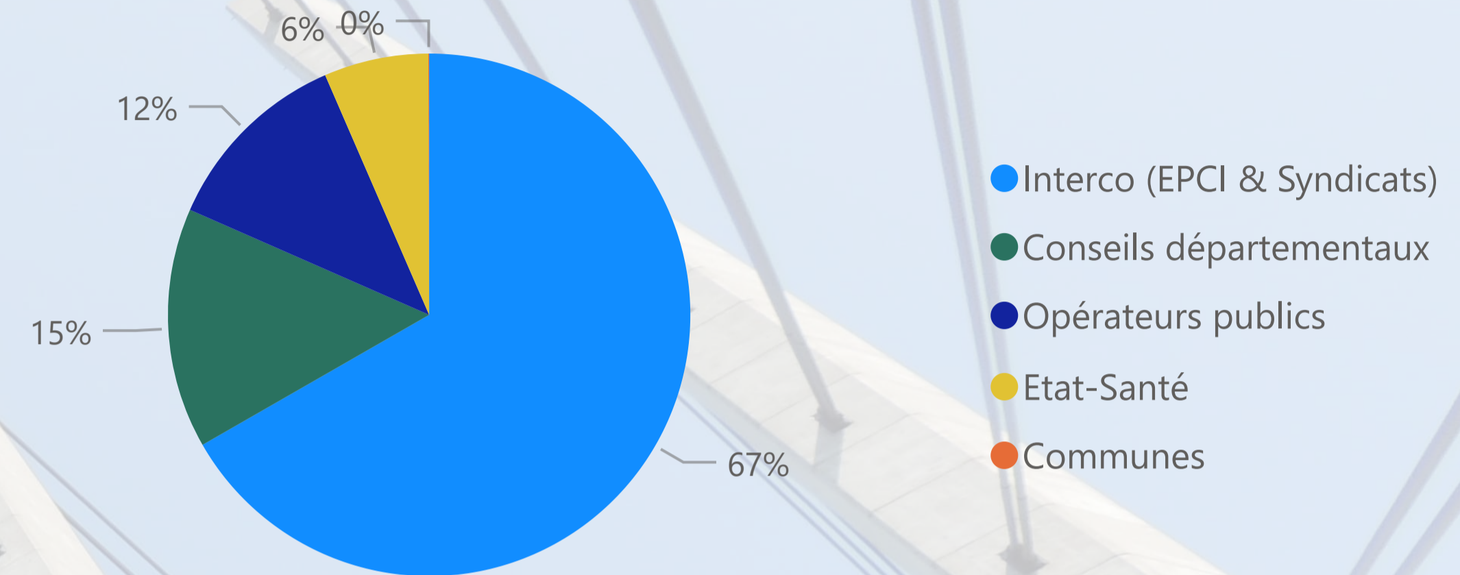
Projets exceptionnels - Répartition des types de MOA
