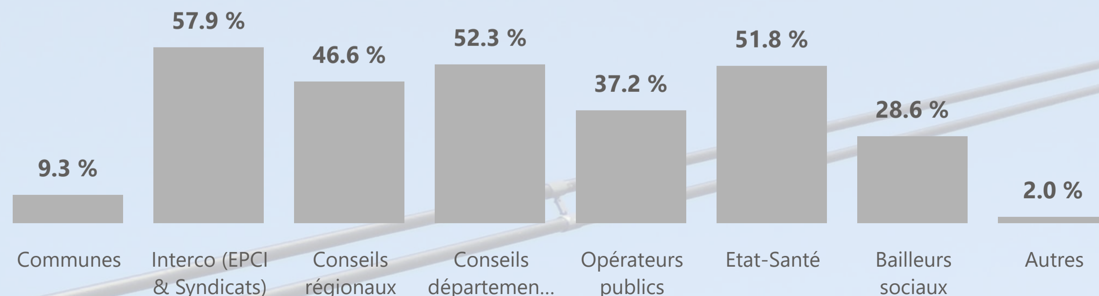
Poids du renouvellement par type de MOA
